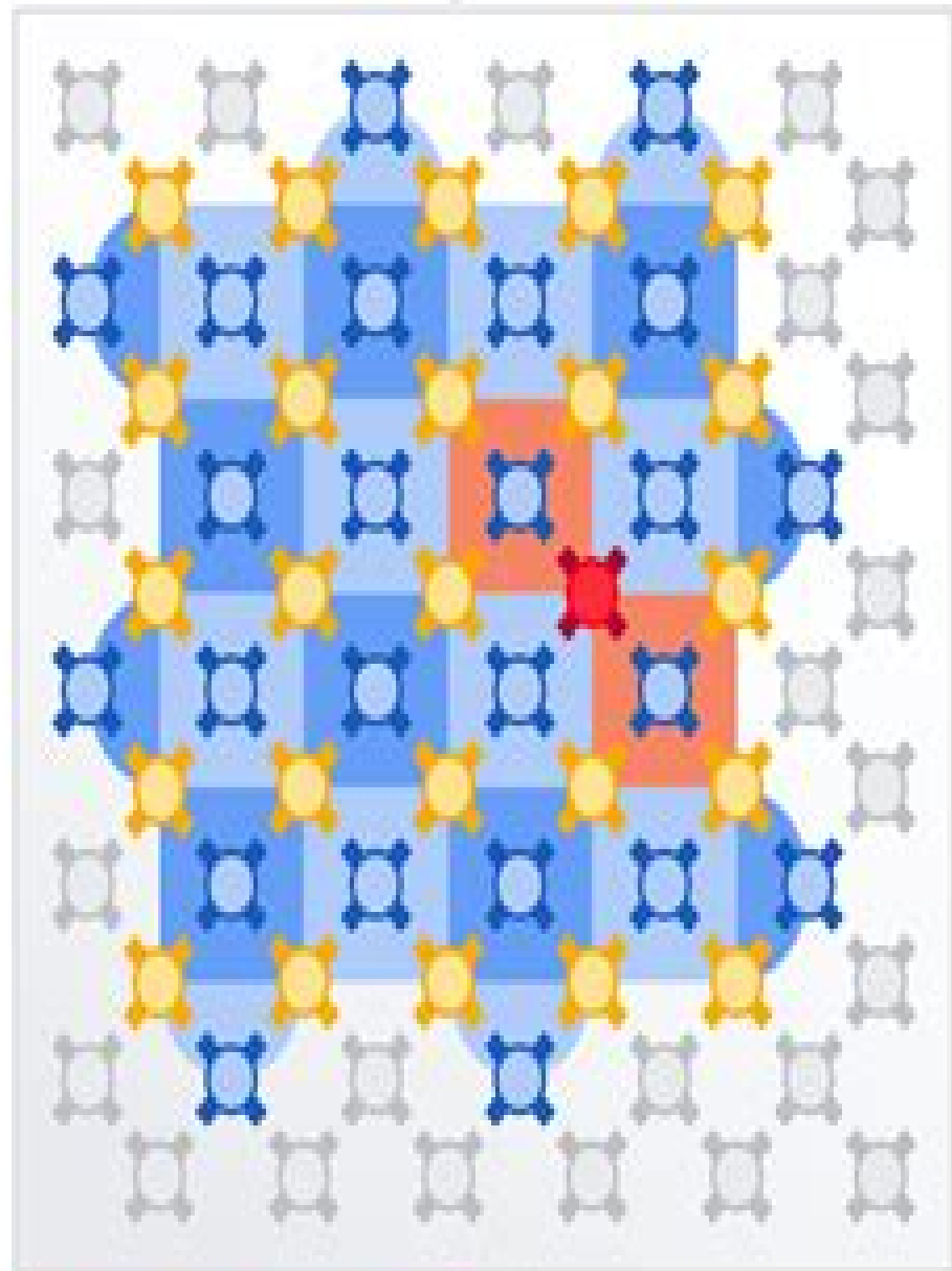
Bit-flip error
