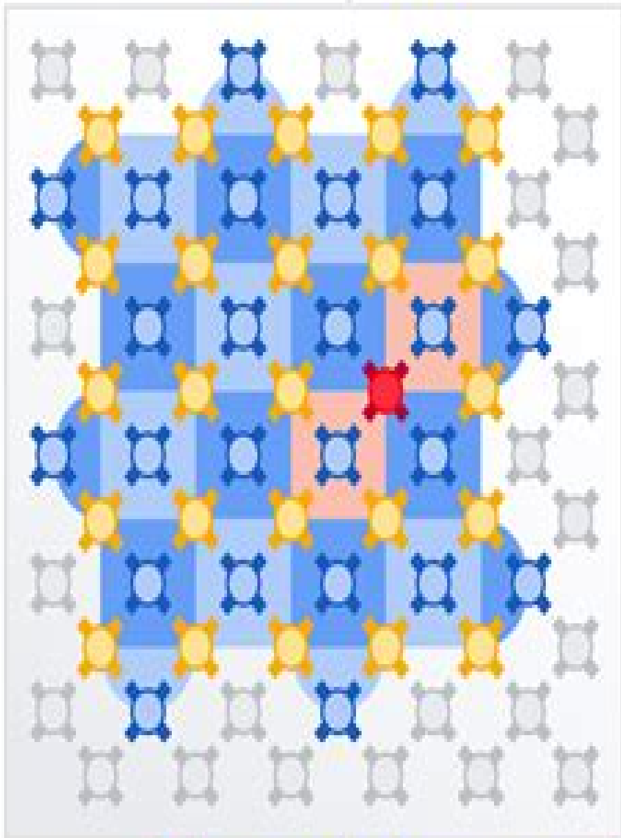
Phase-flip error
