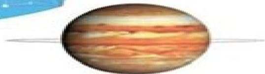
Jupiter
