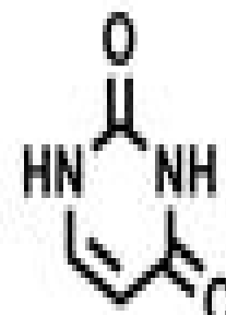
Uracil
