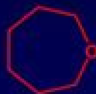
oxepane
