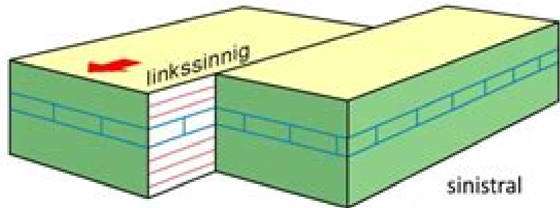
Blattverschiebungen
