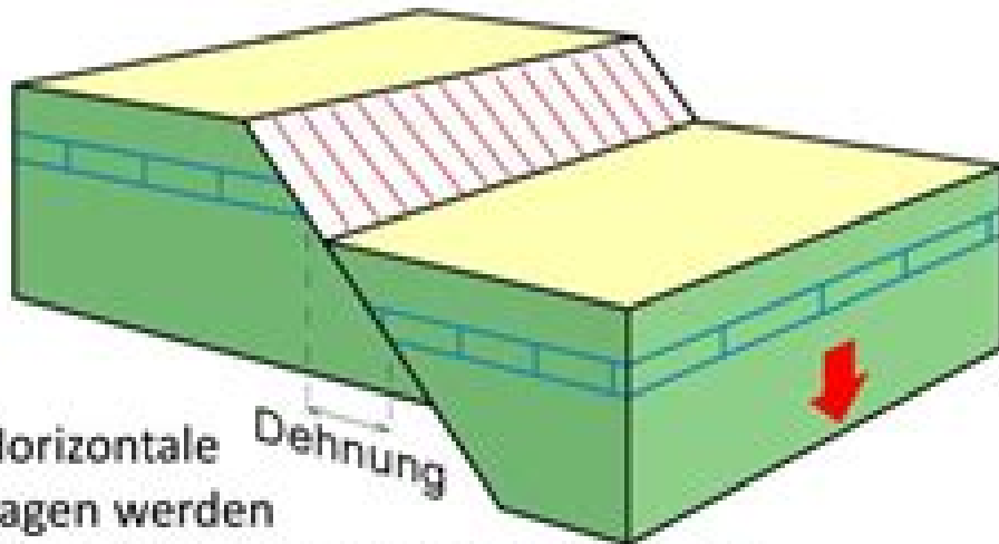
Abschiebung
