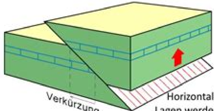
Aufschiebung Überschiebung
