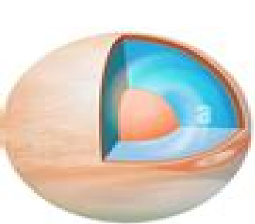
Jupiter
