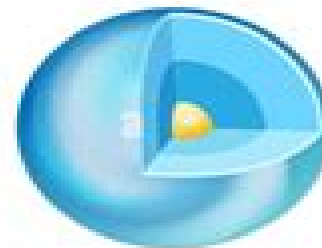
Uranus
