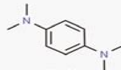
TMPD
