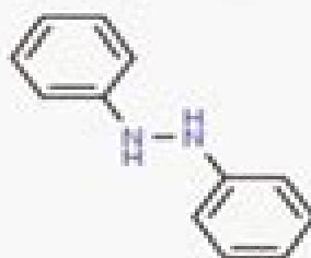
Hydrazobenzene
