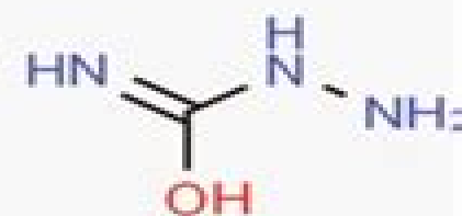
Semicarbazide
