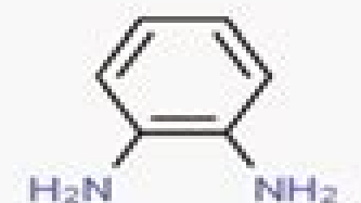
Phenylenediamine
