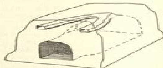
1. Aus Steinen aufgeschichteter Ofen, ohne Bindemittel (fi. kiva ). Der Rauch steigt durch die Ritzen zwischen den Decksteinen auf. Nach Valonen 1963.
