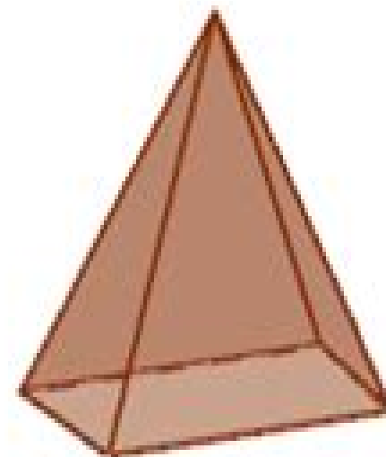
Pyramid
