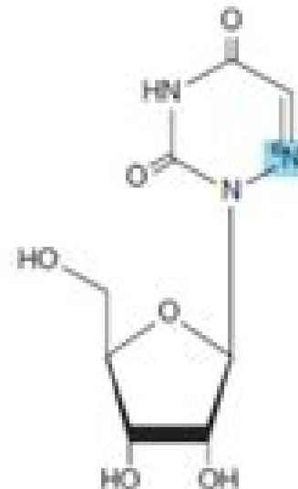
6-Azauridine
