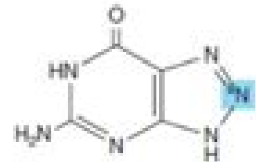
8-Azaguanine
