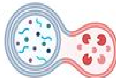
Autophagy
