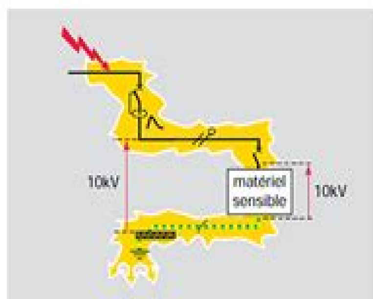
schéma 2 : sans parafoudre, le matériel "claque"
