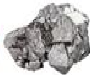
magnetite
