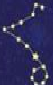
双鱼座 Pisces
