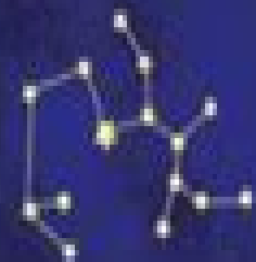
射手座 Sagittarius
