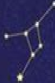
巨蟹座 Cancer
