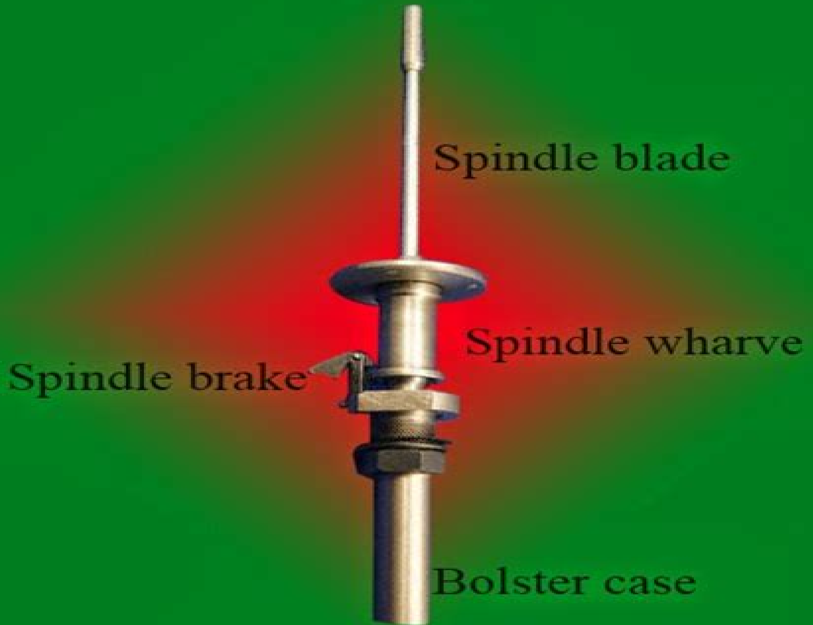
Fig: Spindle
