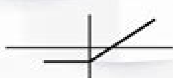
Long Call
