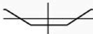
Long Straddle
