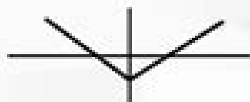
Long Straddle
