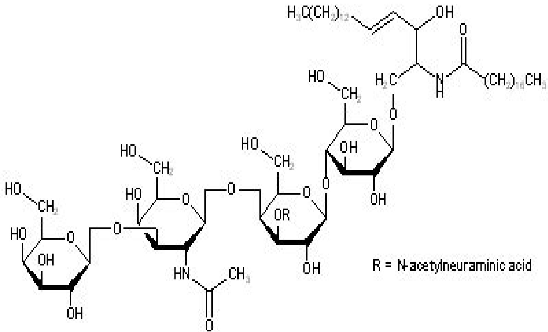
Ganglioside G_{M1}
