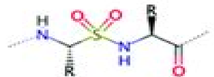
peptidosulfonamides
