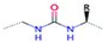
oligourease
