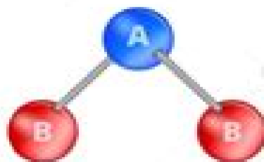
Bent
