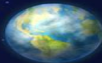
Earth
