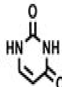
Uracil
