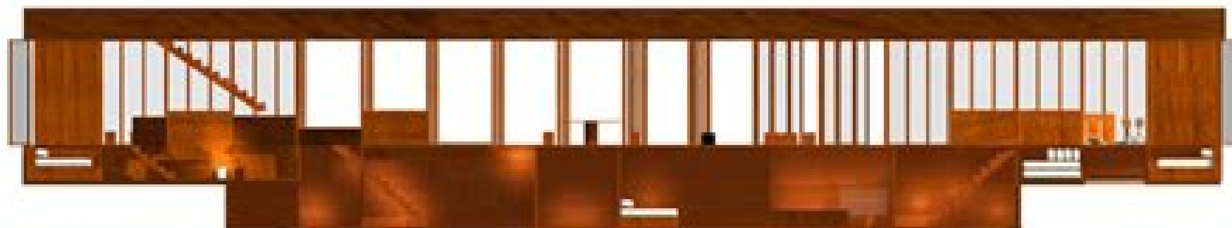
longitudinal section
