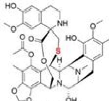
Ecteinascidin 743 (anticancer drug)
