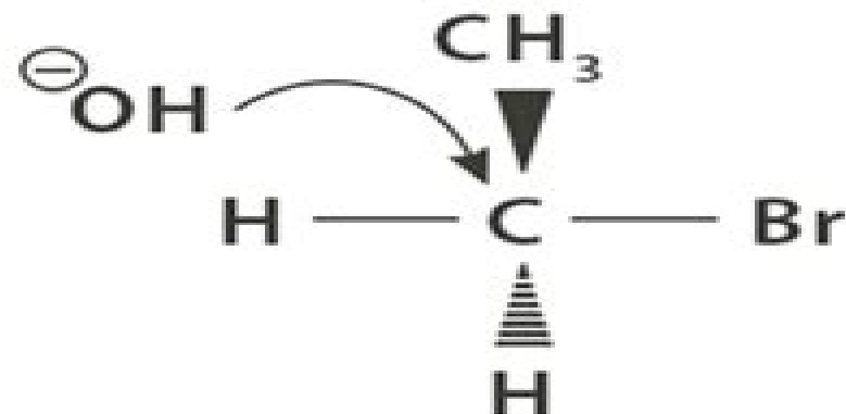
② Ethyl bromide ( 1^\circ carbon)
