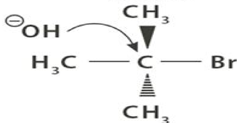
④ tert-Butyl bromide ( 3^\circ carbon)
