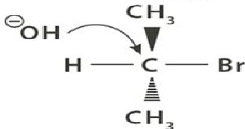
③ Isopropyl bromide ( 2^\circ carbon)
